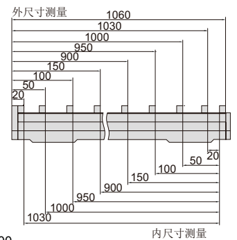
内尺寸测量
