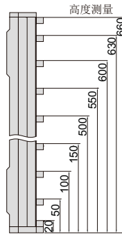
高度测量
