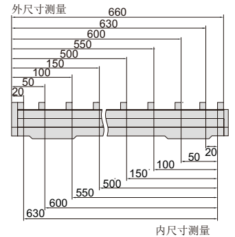
内尺寸测量
